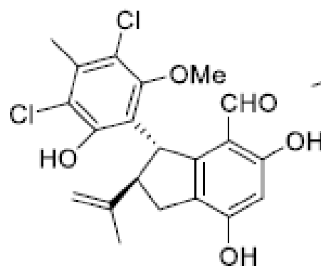
Pestalachloride F
