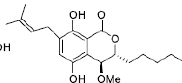
Eurotiumide B
