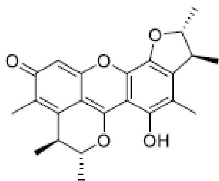
Dicitrinin A
