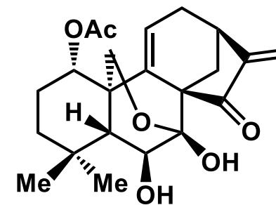
isoadenolin I (6)
