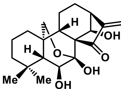
longikaurin A (4)
