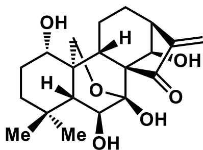
oridonin (1)
